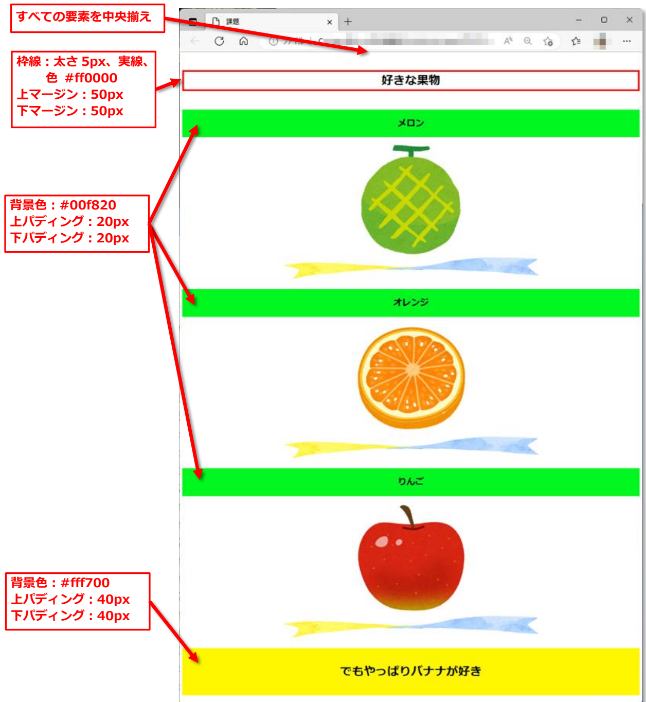
図3 style05.css を適用したページのブラウザ表示
